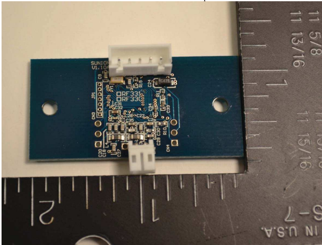
4. RFID PCB Top
