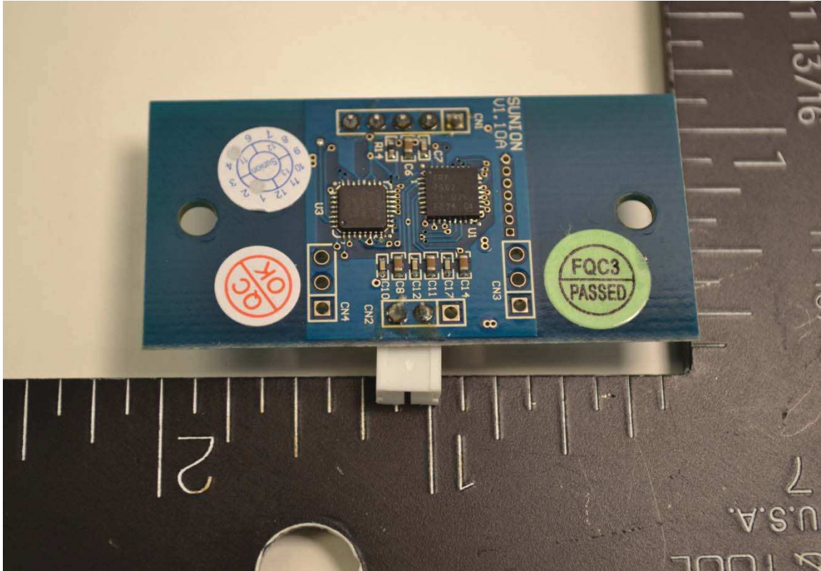
5. RFID PCB Bottom
